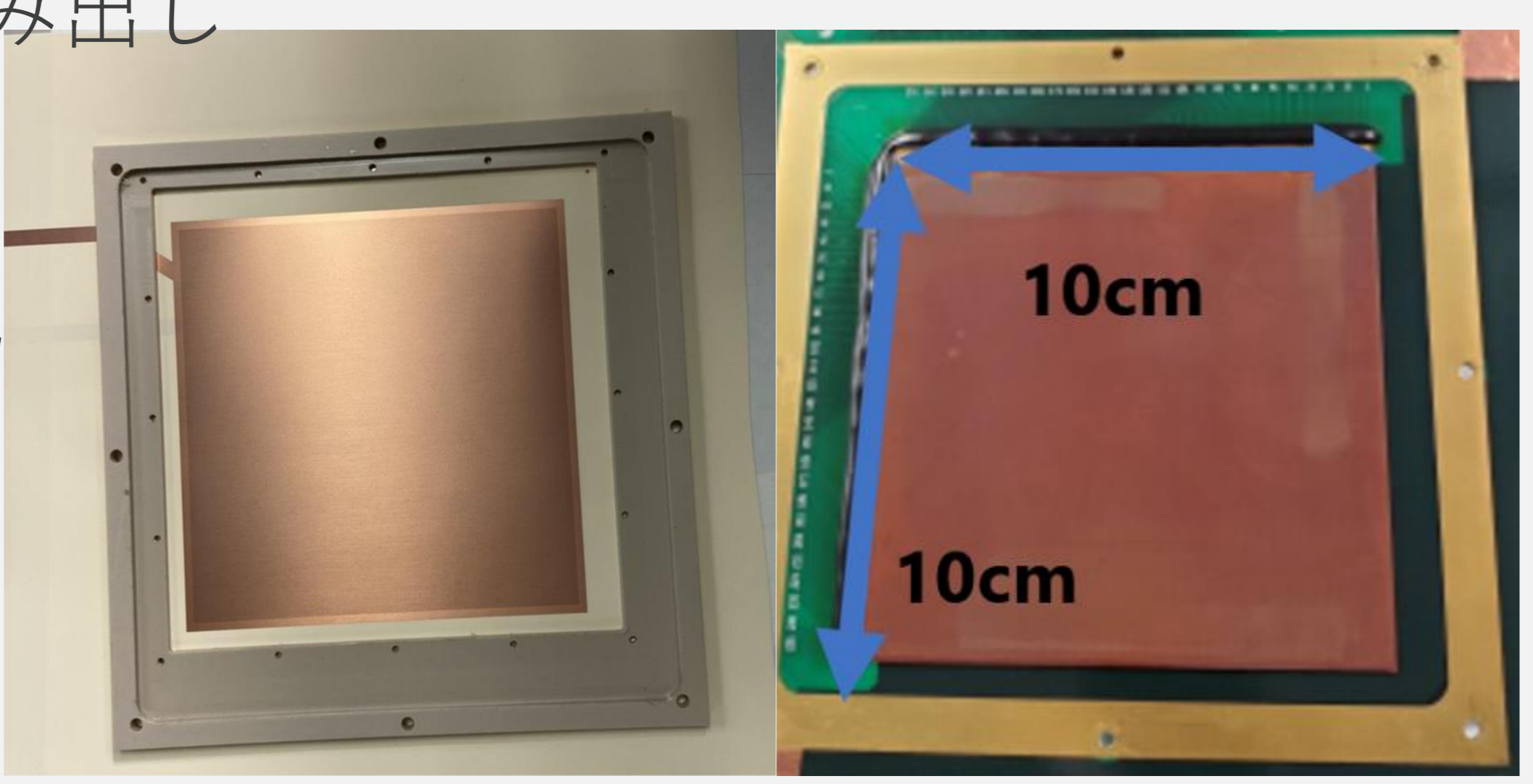
検出器写真 (左：GEM、右：μ-PIC)
