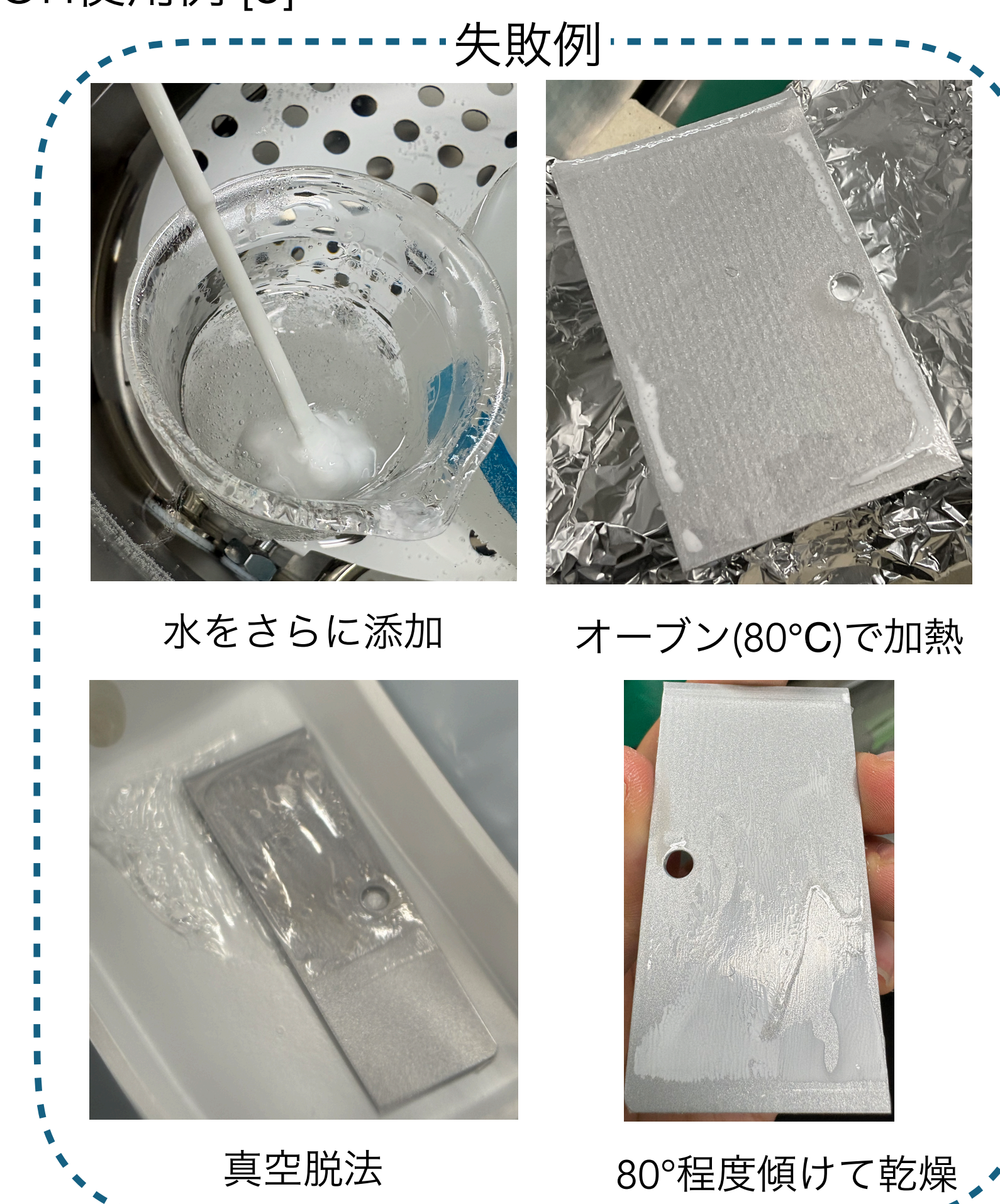
図3. EVOH使用例 [3]
