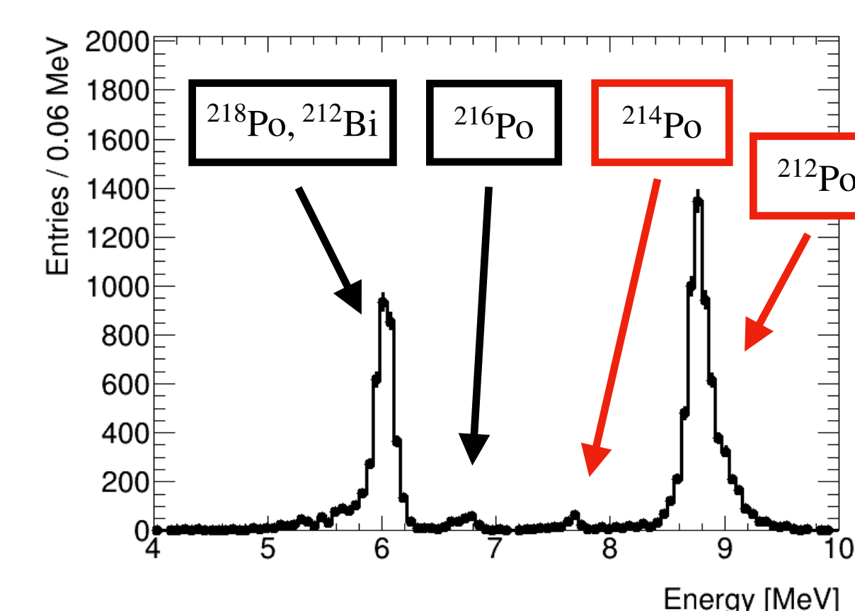
図4. エネルギースペクトル (EVOHなし)
