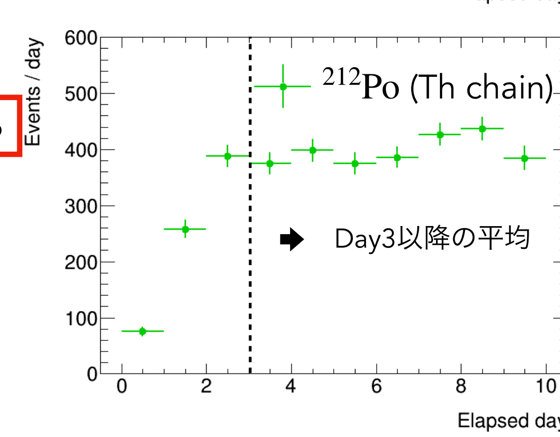
図5. ^{214}\text{Po} , ^{212}\text{Po} レート (EVOHなし)
